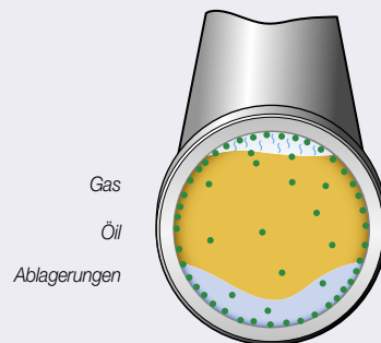
Pipeline Querschnitt der den aktiven VpCI Schutz in der Gasphase, Flüssigkeit und an der Schnittstelle verdeutlicht.
